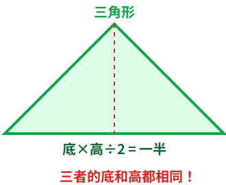
同一底和高下，三個形狀的面積關係
